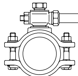
サドル付分水栓 PE一体型
