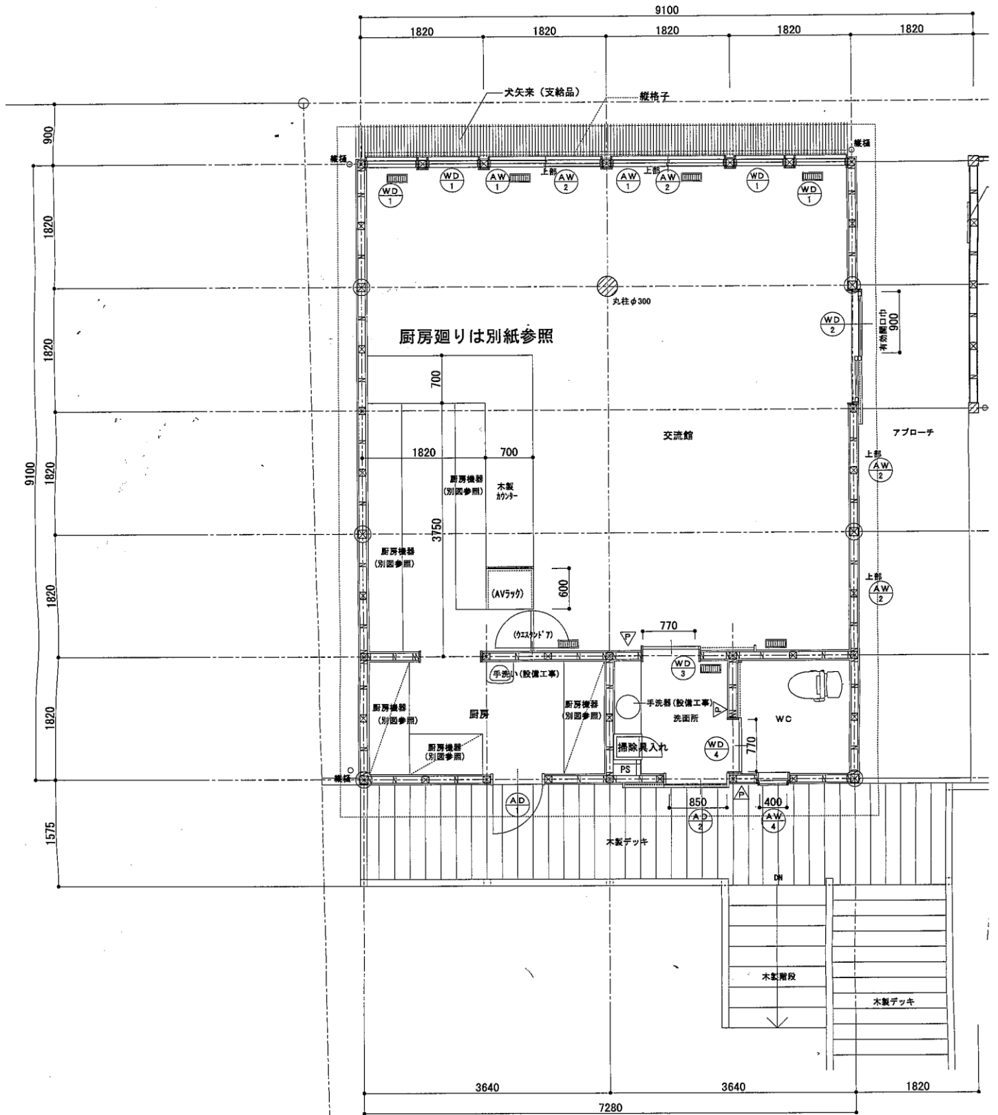
御嶽宿わいわい館茶房棟平面図
