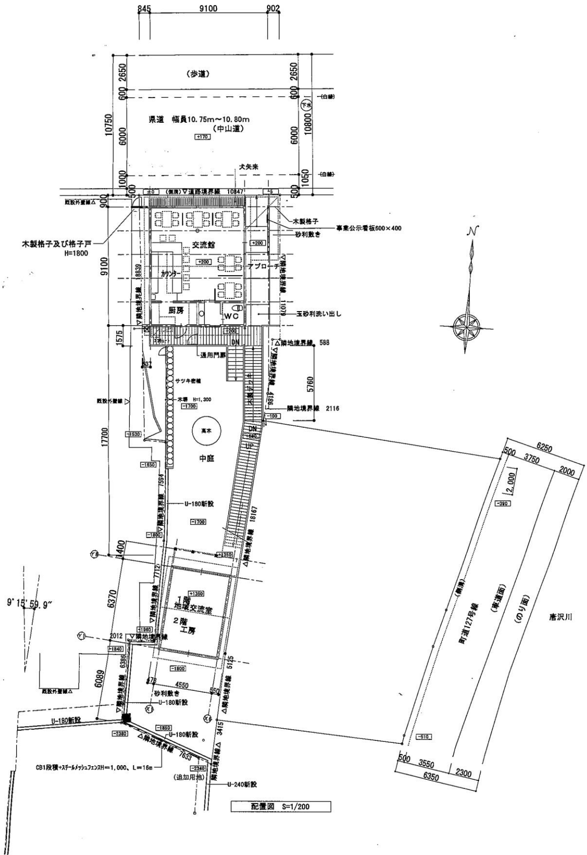
御嶽宿わいわい館配置図
